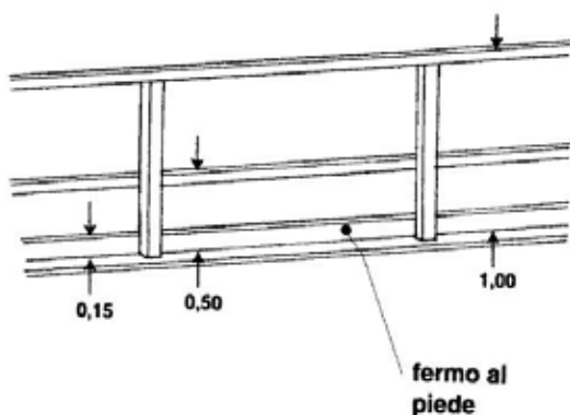
Figura 2 – Parapetto con fermo al piede.
