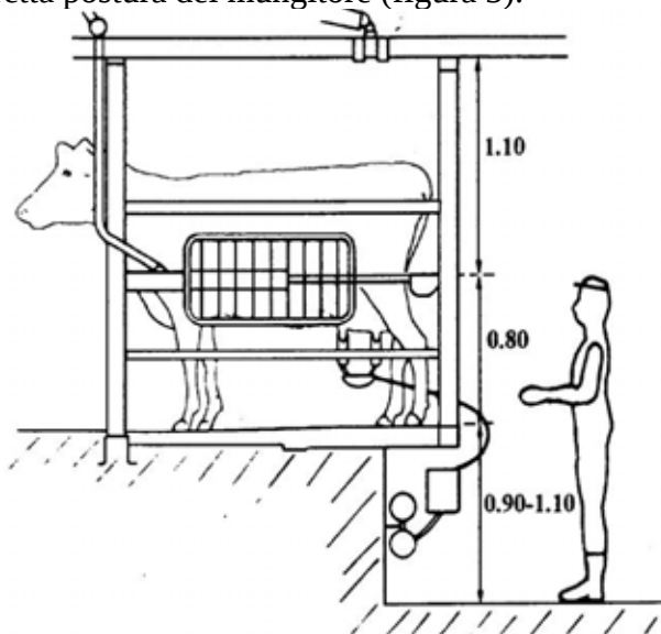
Figura 3 – Il dimensionamento della fossa di mungitura evita l'assunzione di posture errate.
