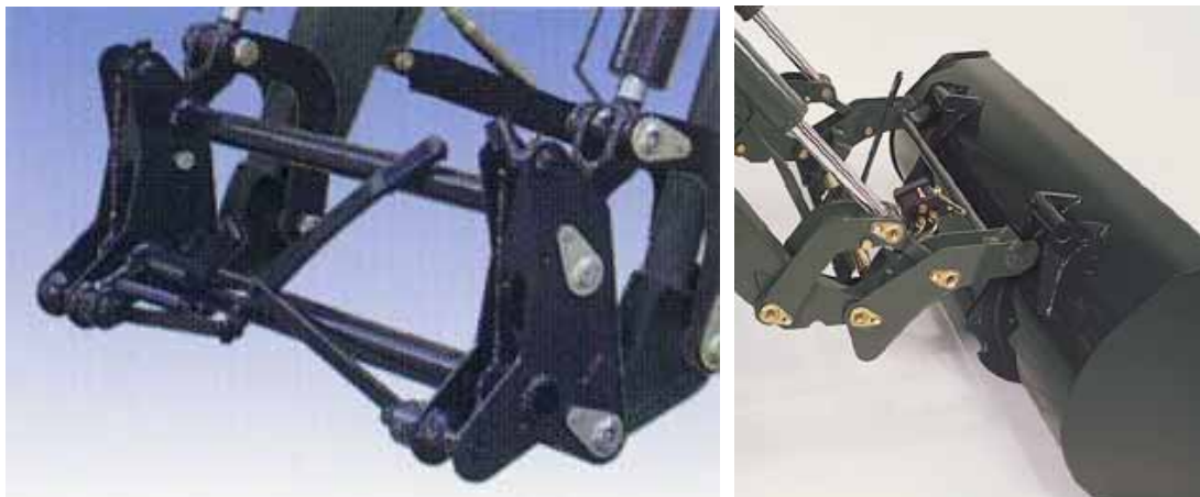
Fig. 2 – Dispositivo di attacco rapido all'estremità dei bracci dei vari attrezzi del caricatore frontale.
