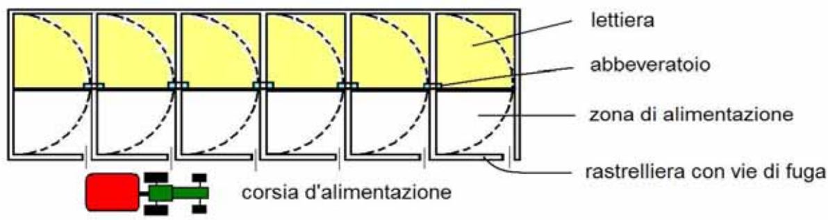
Figura 5 – Stalla con recinti in grado di isolare il gruppo di animali durante le fasi di governo della stalla
