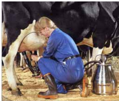
Figura 23 – Gruppo di mungitura a secchio per stabulazione a posta fissa.
