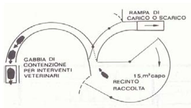
Figura 8 – Sistema per la cattura dei bovini in occasione dei controlli veterinari (Hoenli. 1997).
