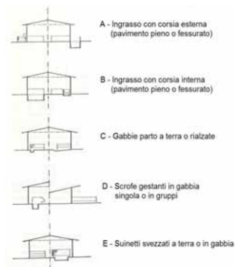
Figura 3 – Sezioni dei principali tipi di porcilaia.
