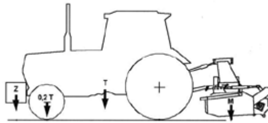
Fig.21 - Per assicurare una reale funzionalità della struttura di sicurezza, non bisogna sovraccaricare il trattore, per non superare il peso proprio oltre a quello massimo ammesso.
