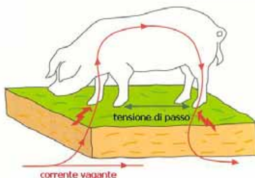
Figura 3 – Tensione di passo.
