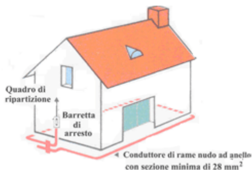
Figura 2 – Anello nel fondo di uno scavo.
