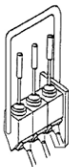
Fig. 3 - Per l'azionamento dei bracci porta fresa e della rotazione della fresa, è necessaria una protezione dinamica dell'operatore mediante dispositivo a "uomo presente" (a sinistra). Inoltre, per evitare pericolosi azionamenti accidentali, il gruppo comandi deve essere idoneamente segregato, ed esempio con un telaio di protezione (a destra).
