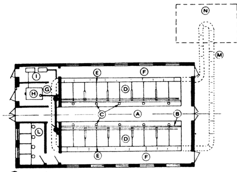
Figura 5 - Pianta orientativa di stalla a posta fissa "testa a testa". A = corsia di alimentazione (larghezza variabile); B = mangiatoia; C = abbeveratoi; D = posta; E = cunetta; F = corsia di servizio; G = impianto di mungitura; H = locale ricevimento latte; I = locale motori, L = locale vitelli; M = nastro trasportatore; N = concimaia a piattaforma (da Hoepli, 1997)
