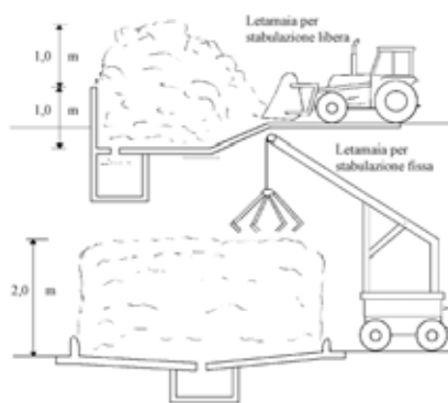
Figura 29 – Letamaie e relative attrezzature di prelievo.
