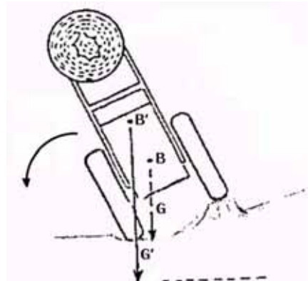
Fig. 10 - Talvolta, anche a causa del carico eccessivo, si possono verificare dei pericolosi sbilanciamenti laterali, in caso di cedimento delle ruote a valle (ad es. per una buca o un avallamento) e/o interferenza di una cunetta con quelle a monte.
