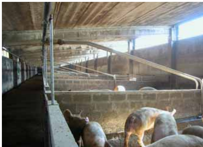
Figura 15 – Valvole di distributore del pastone.
