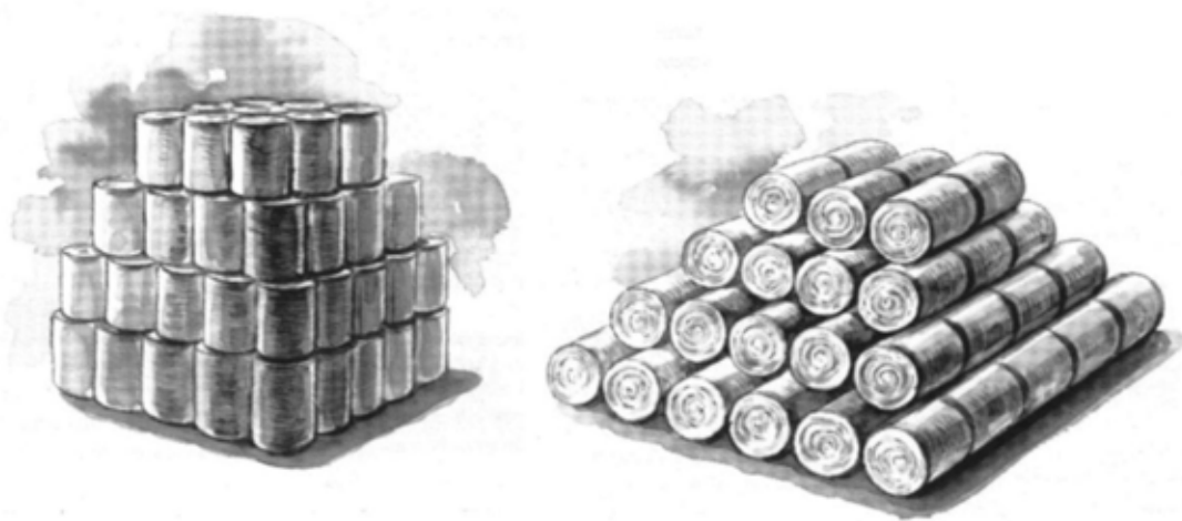
Figura 6 – Esempi di corretto accatastamento di rotoballe (a sinistra con blocchi alla base).
