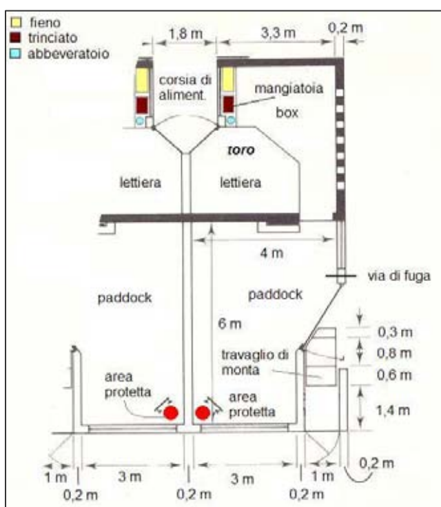
Figura 1 - Schema di recinto ideale per tori (Sainsbury, 1988).
