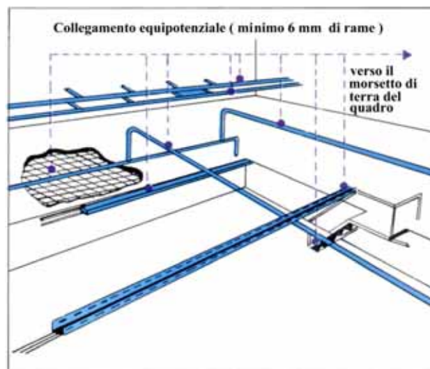
Figura 1 – Esempio di collegamento equipotenziale in sala di mungitura.
